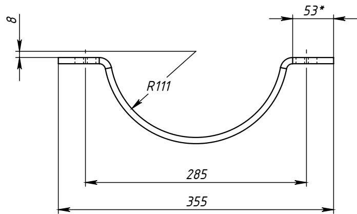
Поз.1 (Полухомут)
