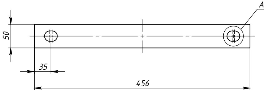
Поз.1 (Полухомут) развертка
