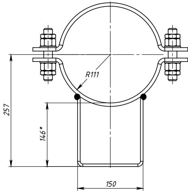
Поз.1 (Полухомут)
